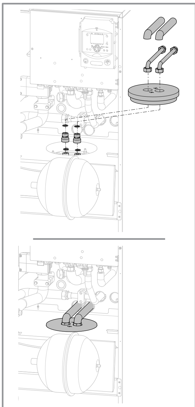
figure 25 - Montage des tuyauterie ECS
