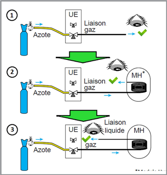
figure 19 - Vérification des liaisons frigorifiques
