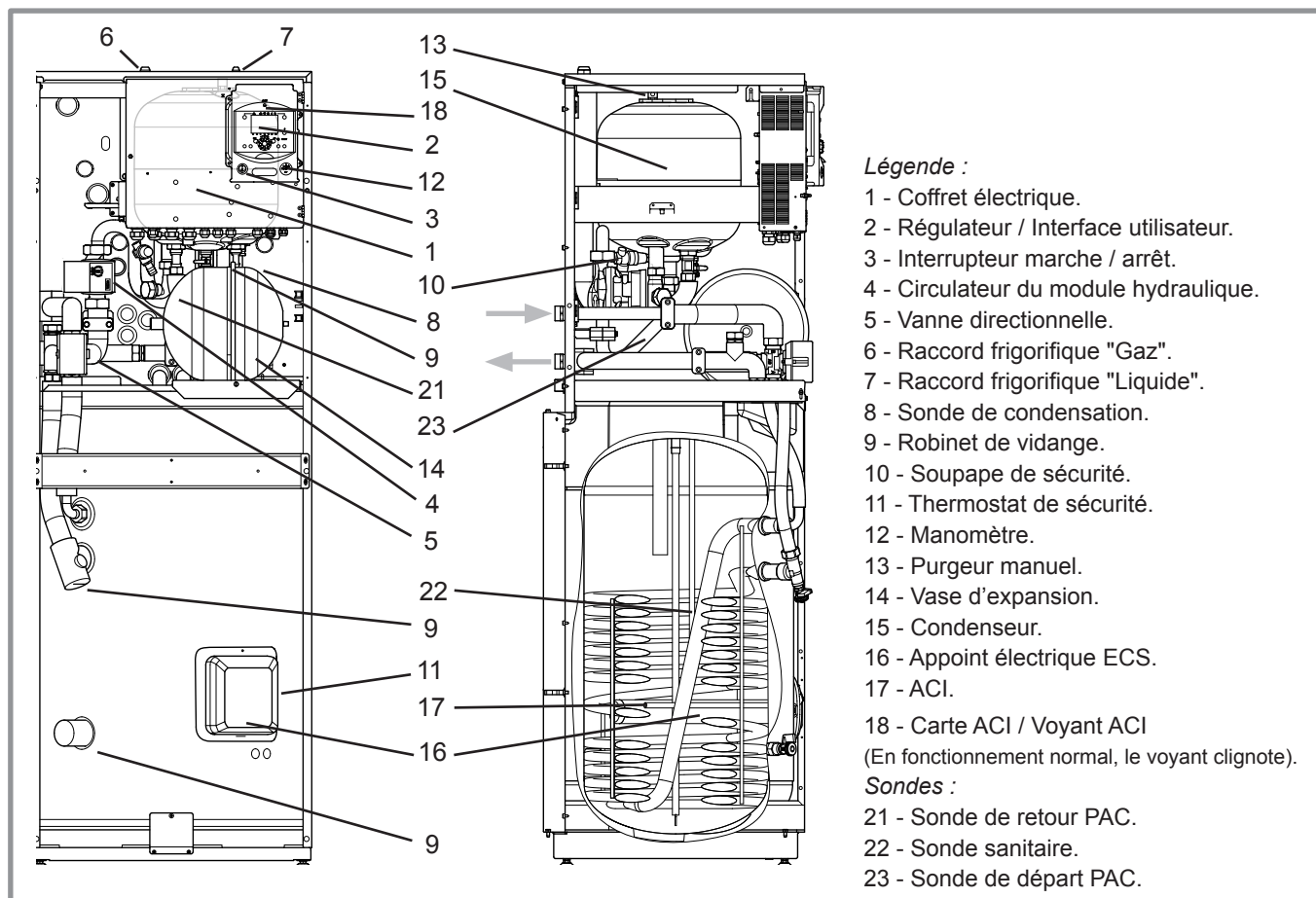
figure 7 - Organes du module hydraulique
