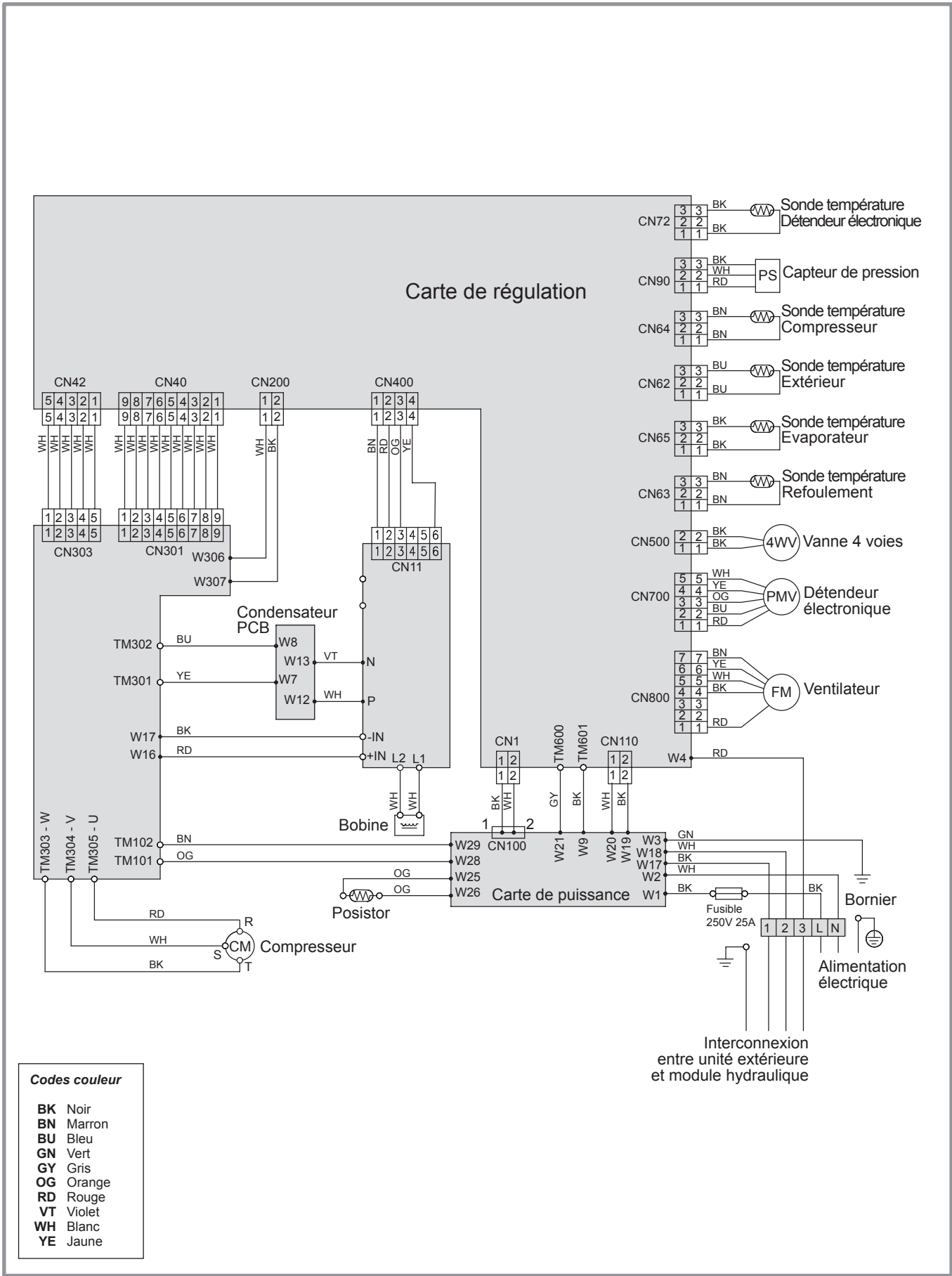
figure 48 - Câblage électrique unité extérieure modèle extensa duo + 10
