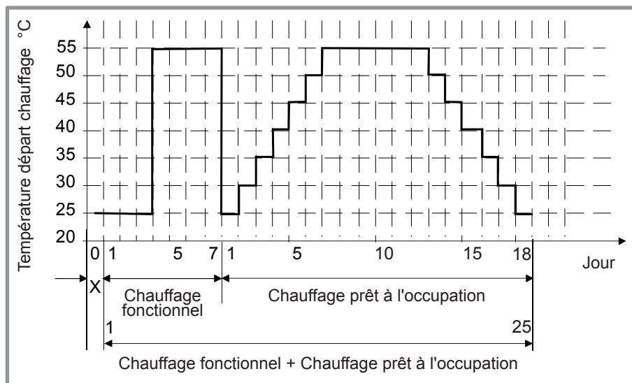
figure 45 - Diagramme des programmes de séchage de dalle
