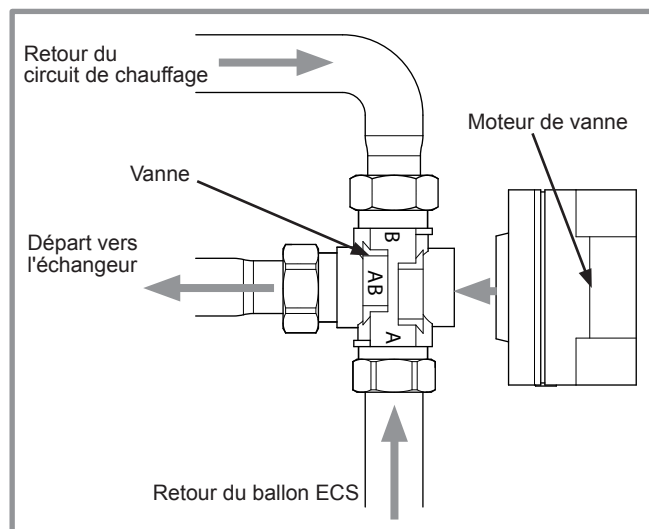
figure 51 - Montage de la vanne directionnelle
