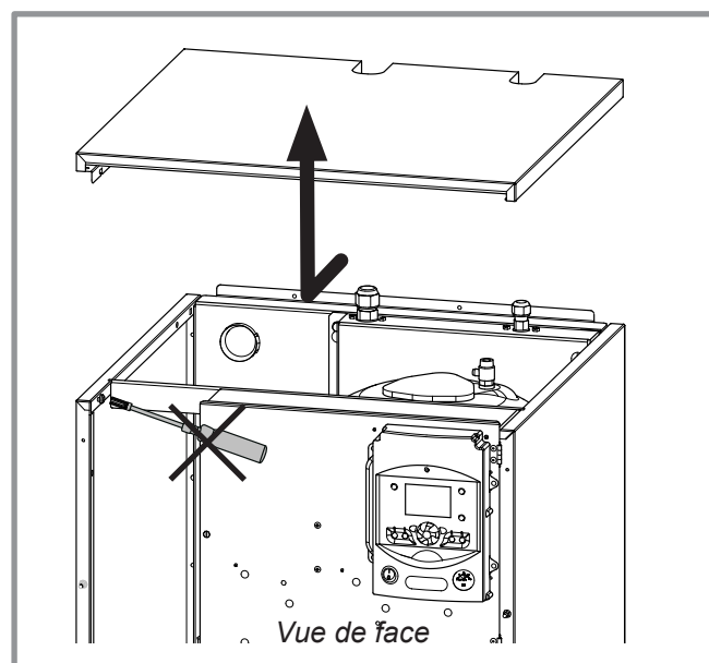
figure 16 - Dépose du couvercle
