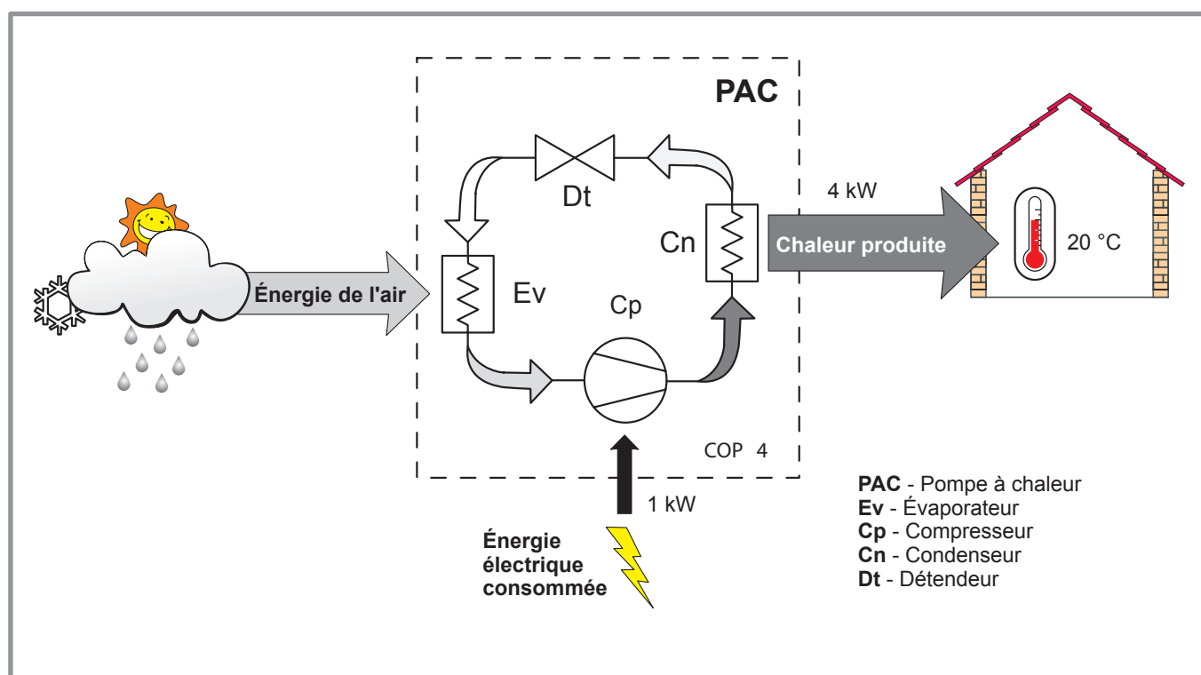
figure 8 - Principe de fonctionnement d'une pompe à chaleur
