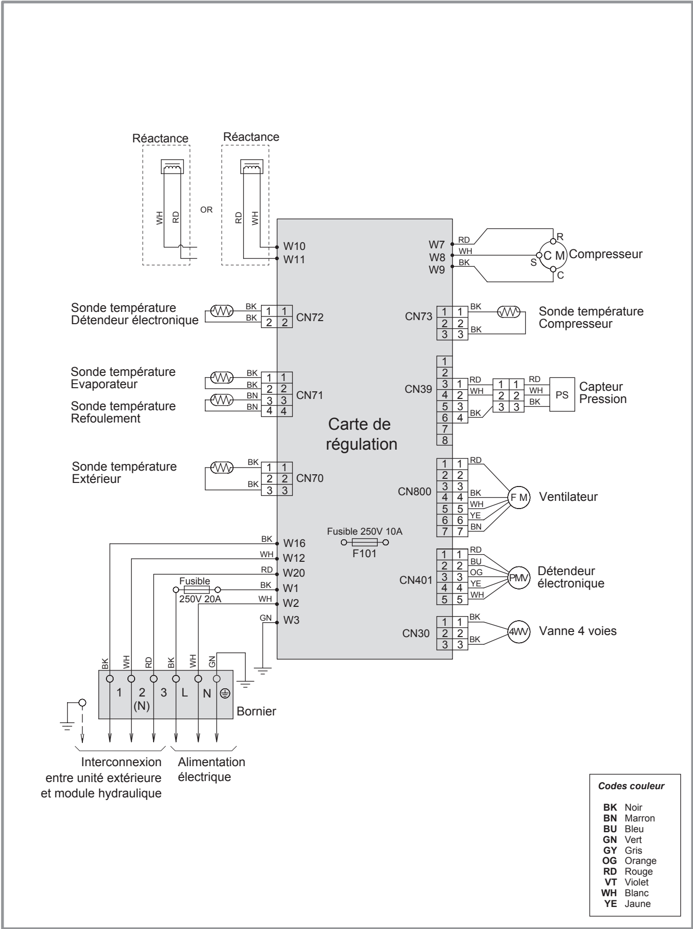
figure 46 - Câblage électrique unité extérieure modèle extensa duo + 5 et 6
