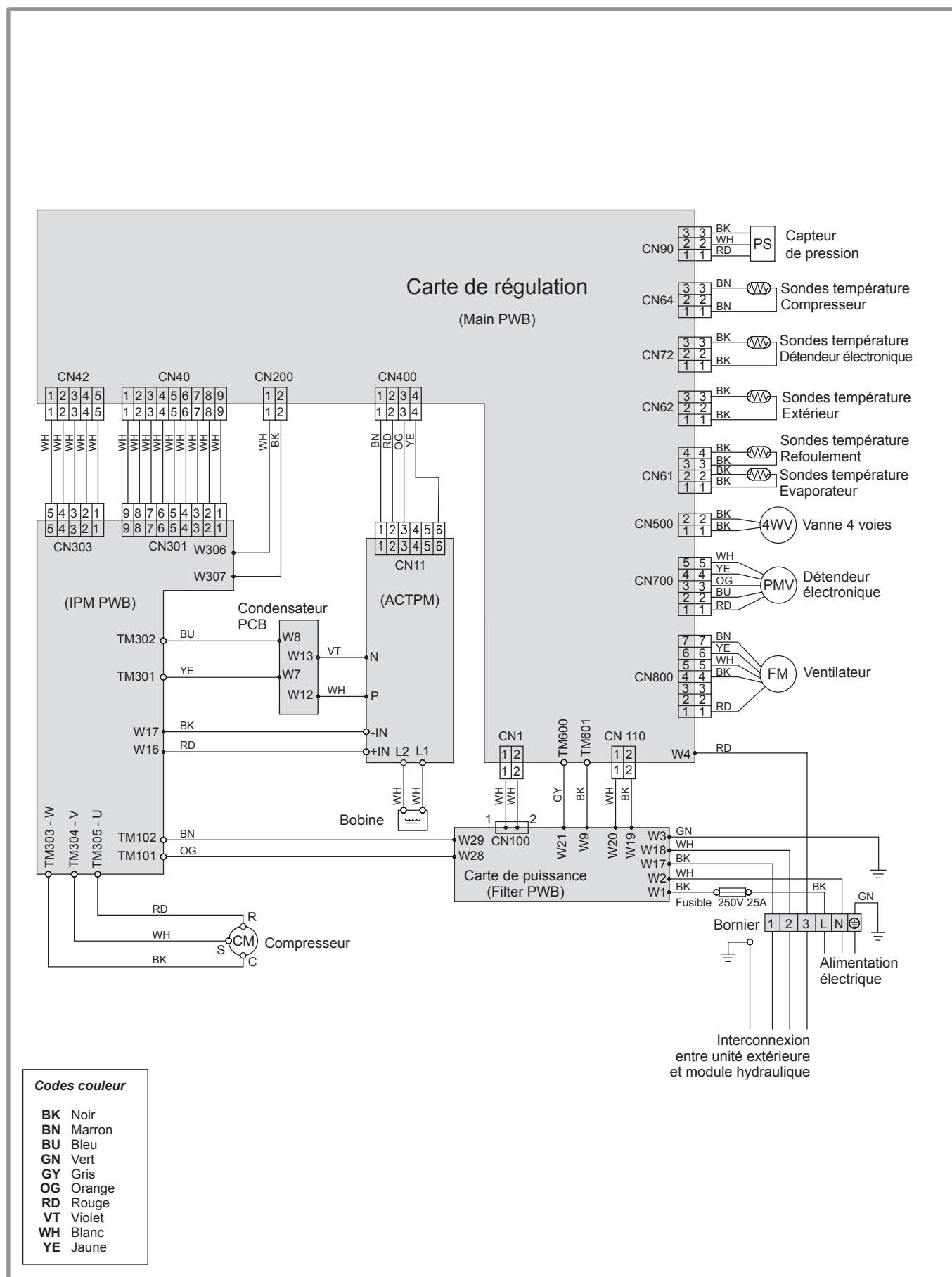
figure 47 - Câblage électrique unité extérieure modèle extensa duo + 8
