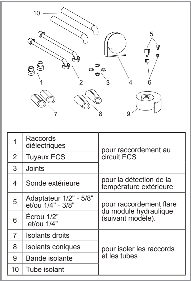
figure 10 - Accessoires fournis avec le module hydraulique
