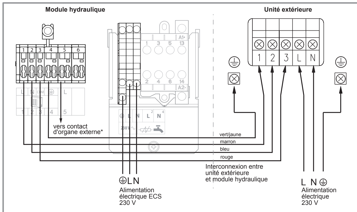
figure 37 - Raccordement aux borniers et relais de puissance
