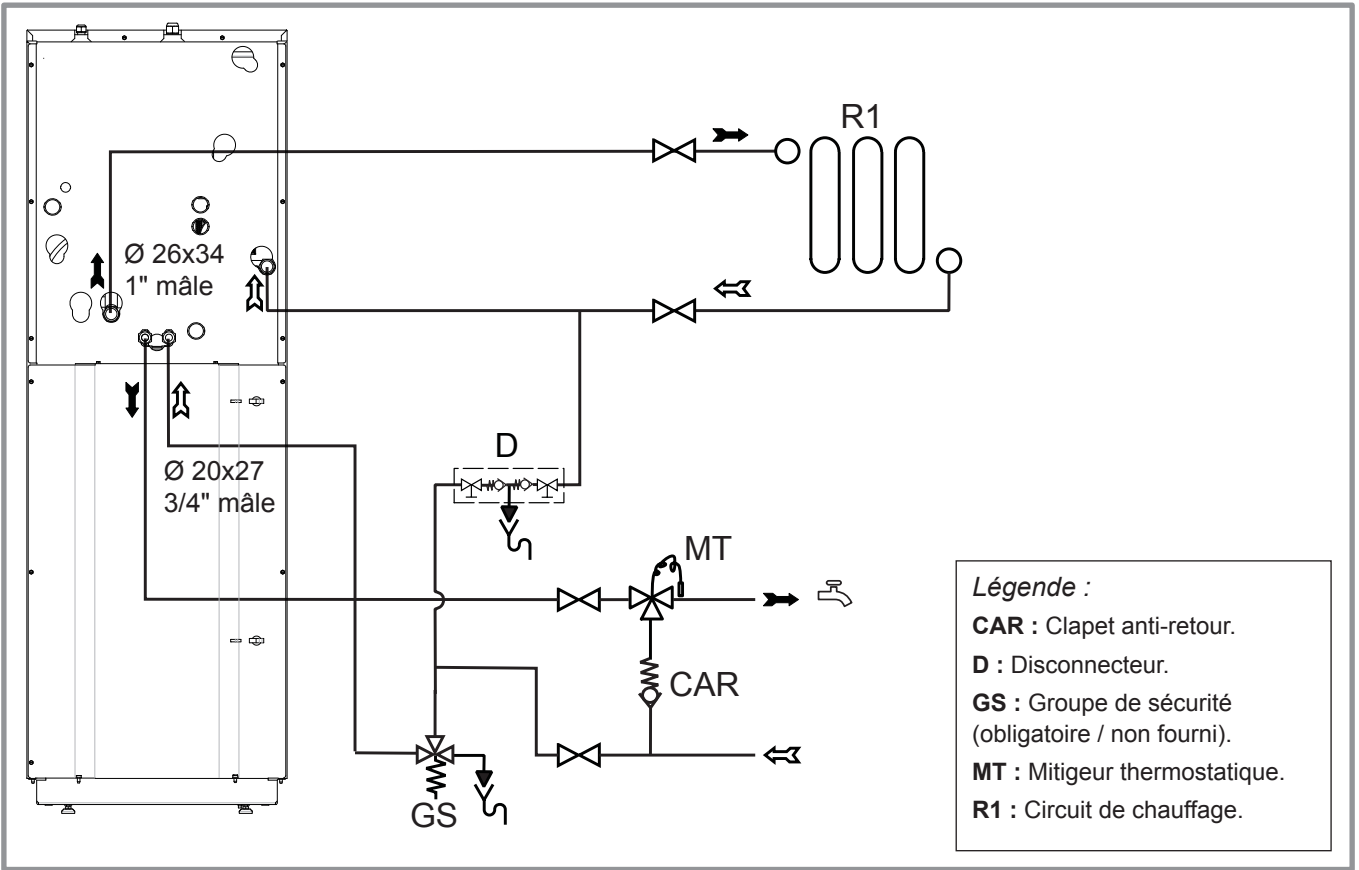
figure 24 - Schéma hydraulique de principe
