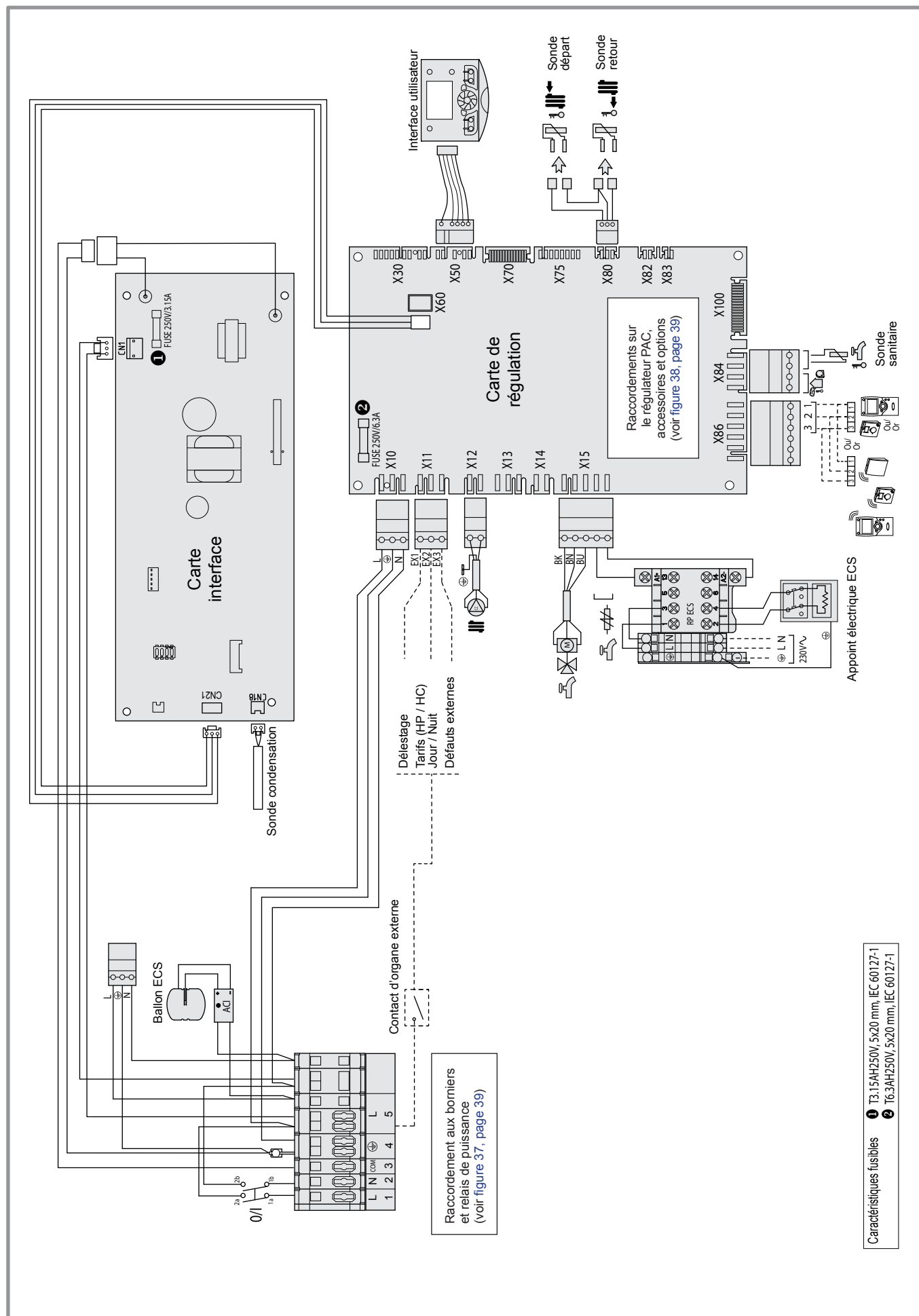
figure 49 - Câblage électrique module hydraulique (hors raccordements installateur)
