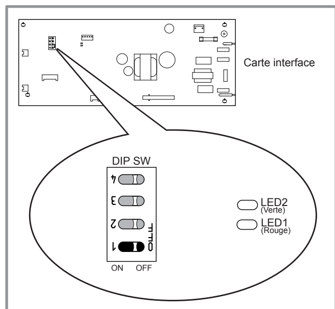
figure 23 - Emplacement des interrupteurs DIP et des LED sur la carte d'interface du module hydraulique
