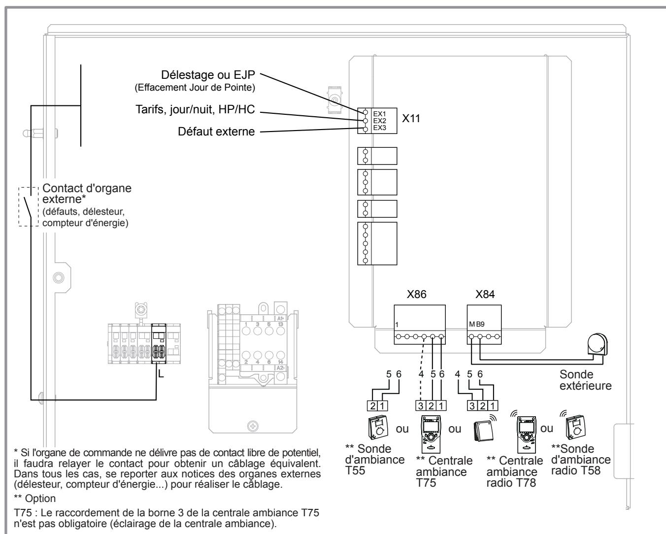
figure 38 - Raccordements sur le régulateur PAC (accessoires et options)
