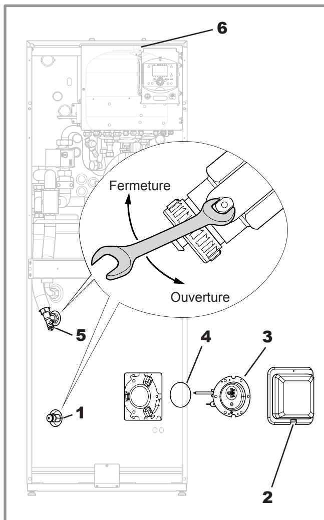
figure 50 - Vidange du module hydraulique et/ou du ballon sanitaire
