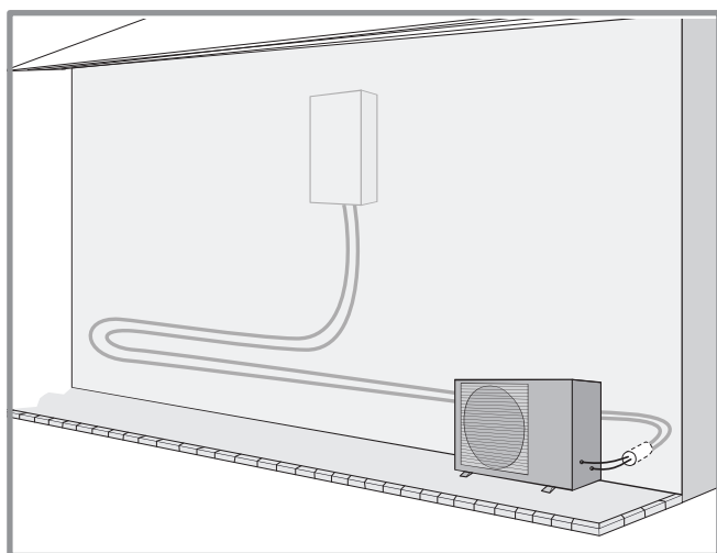
figure 11 - Exemple conseillé de disposition des liaisons frigorifiques
